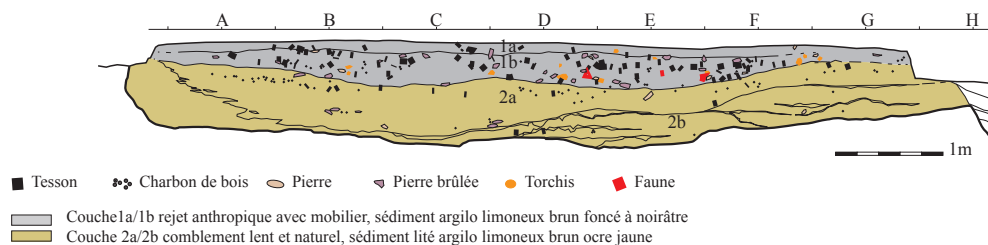
Fig. 3 - Épannes, Les Jardins de Ribray (Deux-Sèvres). Coupe stratigraphique de la fosse polylobée (DAO S. Vacher, Inrap).
