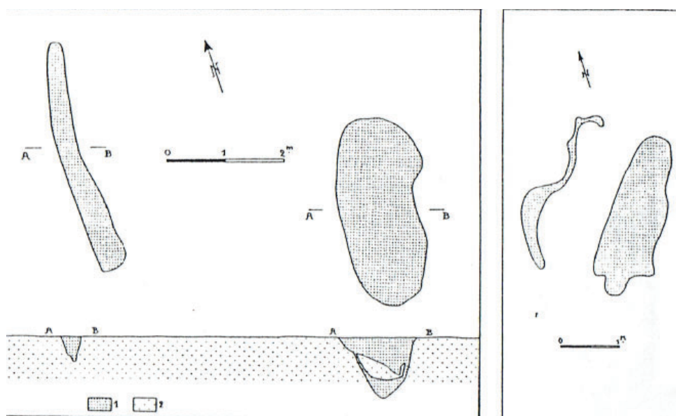
Fig. 10 : Plans et sections de fosses à foyers du Curnic. En pointillé serré, le remplissage riche en charbons de bois ; en blanc sur les plans, et en pointillé lâche sur les coupes, le limon loessique du substratum. A gauche, les deux fosses dégagées lors des fouilles de 1962 ; à droite une fosse vue en 1963.
