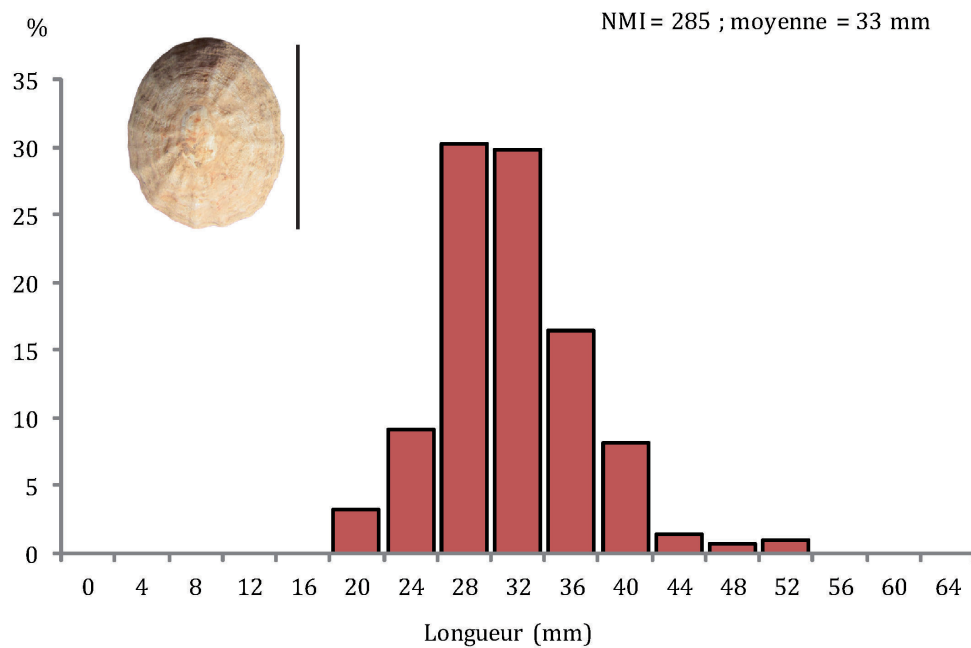
Fig. 14 - Distribution des longueurs des patelles Patella sp. de Mez Notariou pour les niveaux du Bronze moyen.
