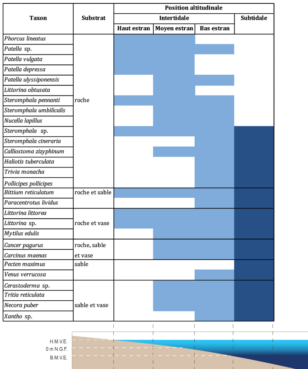
Fig. 22 - Position altitudinale et biotope des invertébrés marins identifiés à Mez Notariou (H.M.V.E. : Haute Mer de Vive Eau ; N.G.F. : Nivellement Géographique de la France ; B.M.V.E. : Basse Mer de Vive Eau, d'après Dupont, 2006).
