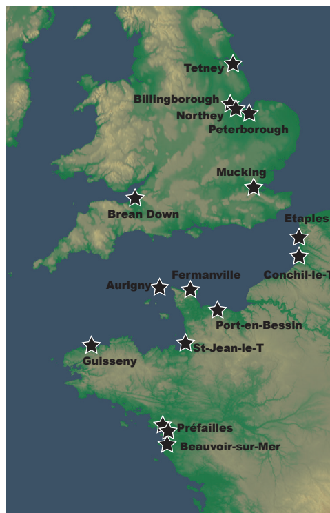
Fig. 1 – Localisation des sites cités dans le texte (DAO C. Marcigny, Inrap).
