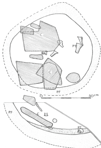
Fig. 10. — Plan et section du four de L'Épinette (Préfailles, L.-A.). PF : parois de la fosse ; C : pierres de couverture ; PT : piliers en trompette.
