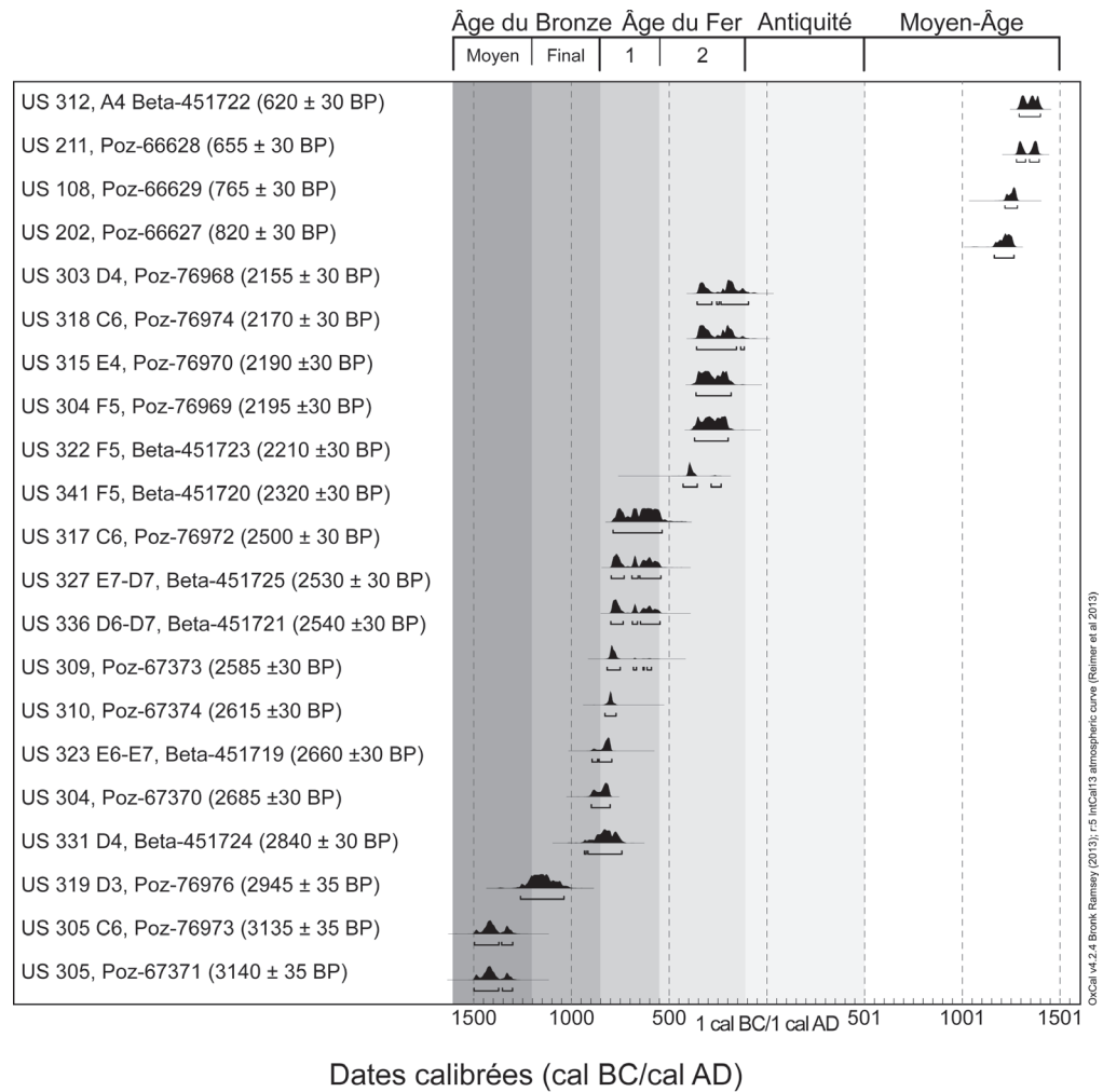
Fig. 3 – I Casteddi : datations calibrées à 2 sigma (DAO : H. Paolini-Saez, X. Villat).
