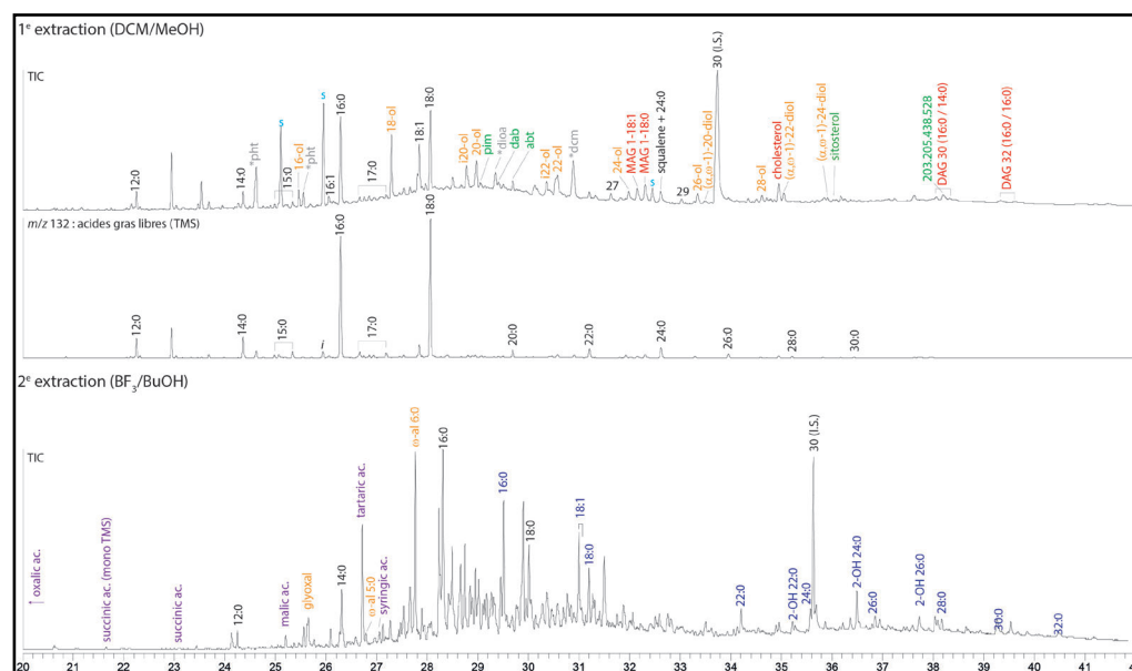
Fig. 7 - Vienne-en-Val « Les Terres de Saint-Germain ». Chromatogrammes du premier et du second extrait obtenus à partir des imprégnations des parois internes de la jatte 2 (extraits triméthylsilylés, analyse GC-MS, colonne Zebron 5MSi 18 m x 0.18 mm d.i. x 0.1 µm ép, détection EI 70 eV) (© N. Garnier, LNG).
